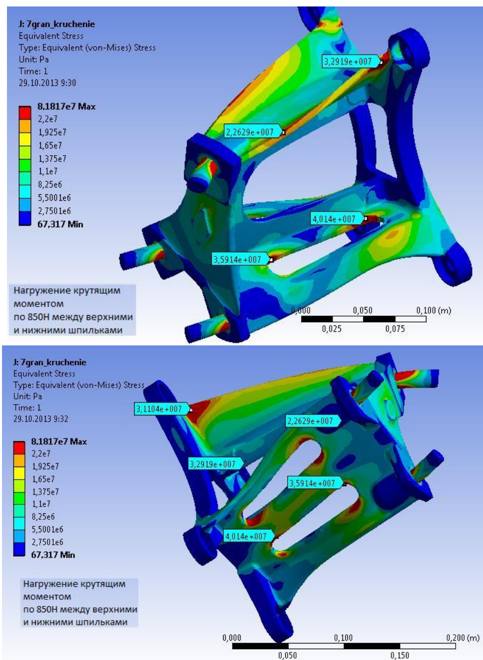
Рис. 1 Прочностные характеристики существующего кронштейна крепления запасного колеса
